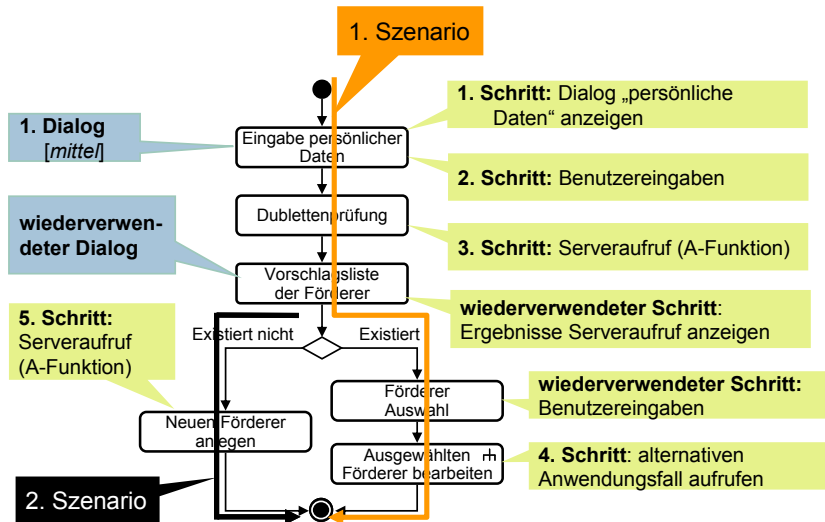
Abbildung 53: Zählung für Use Case „Persönliche Daten anlegen“
