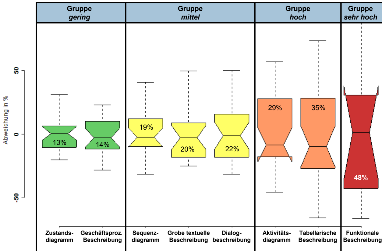
Abbildung 38: Boxplots der transformierten tUCP Schätzreihen als Abweichung vom Mittelwert in Prozent. Der Variationskoeffizient ist in den Boxen als Prozentwert angegeben.
