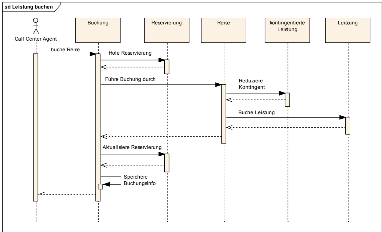
Abbildung 30: Beispiel für ein Sequenzdiagramm
